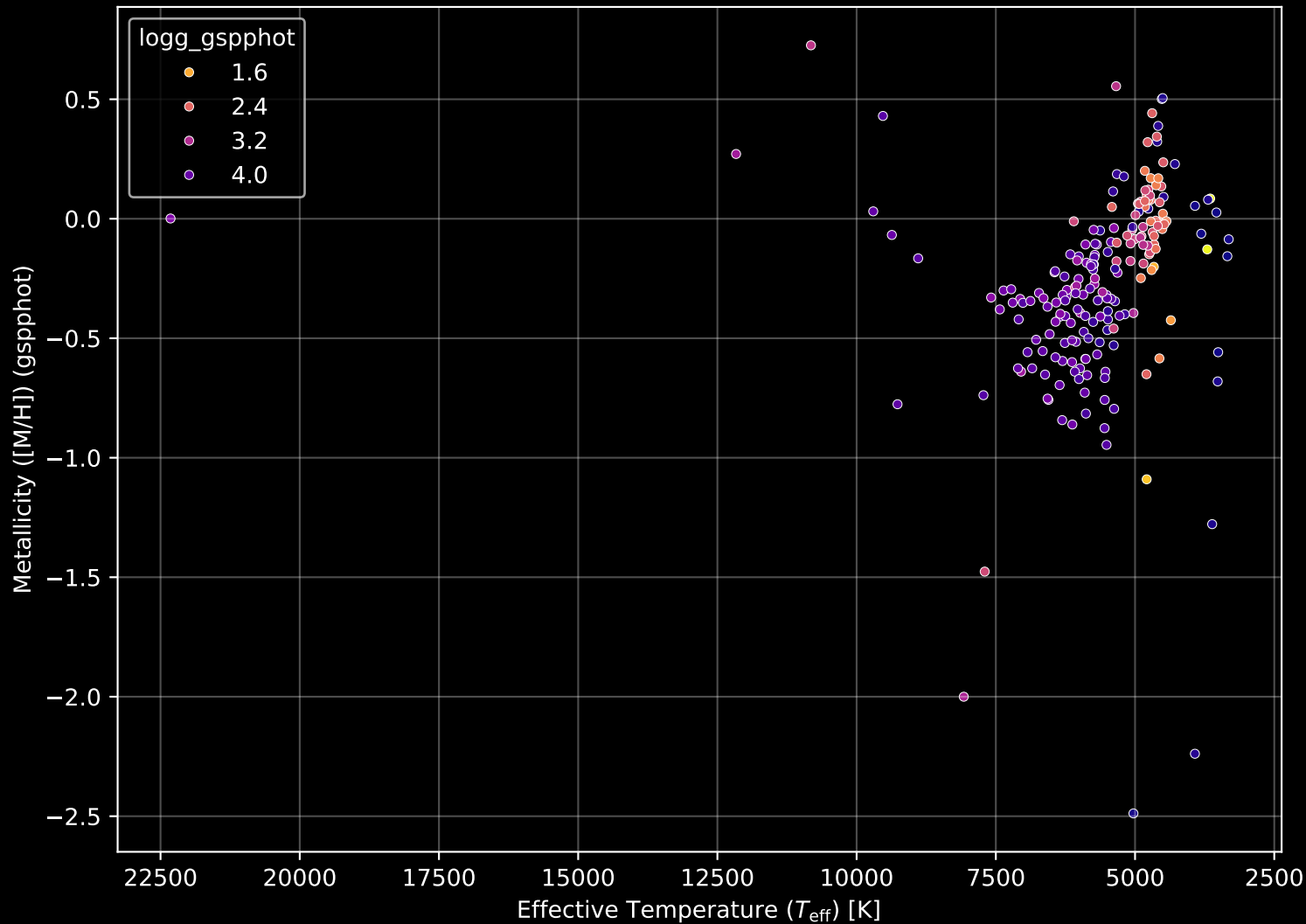
APOGEE DR17 Field: [K2_C7_012-08_btx] Stellar Population Parameters (n= 208)
